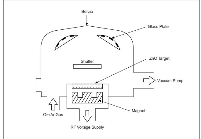
Fig.5 Sputtering apparatus
