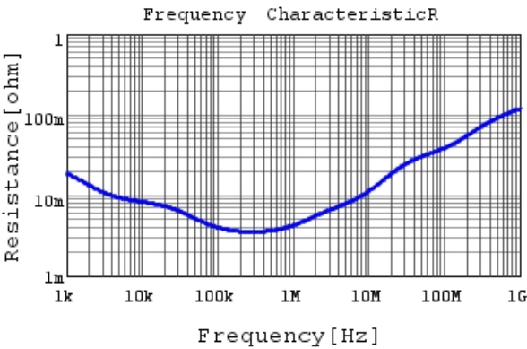
ECASD40E477M006KA0 R DCOV, 25degC
