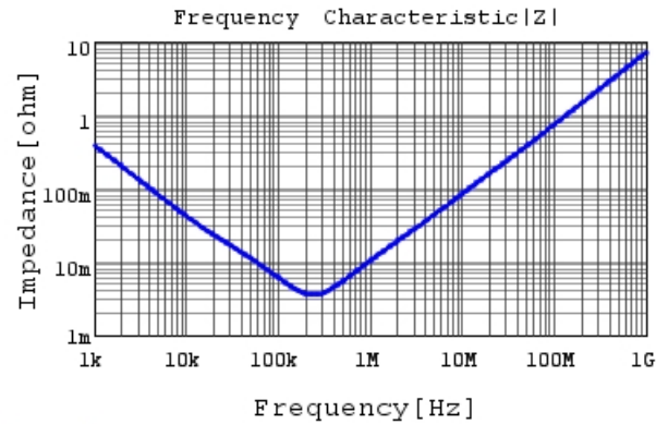
ECASD40E477M006KA0 |Z| DCOV, 25degC
