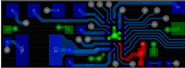
Figure 45. Top Layer
