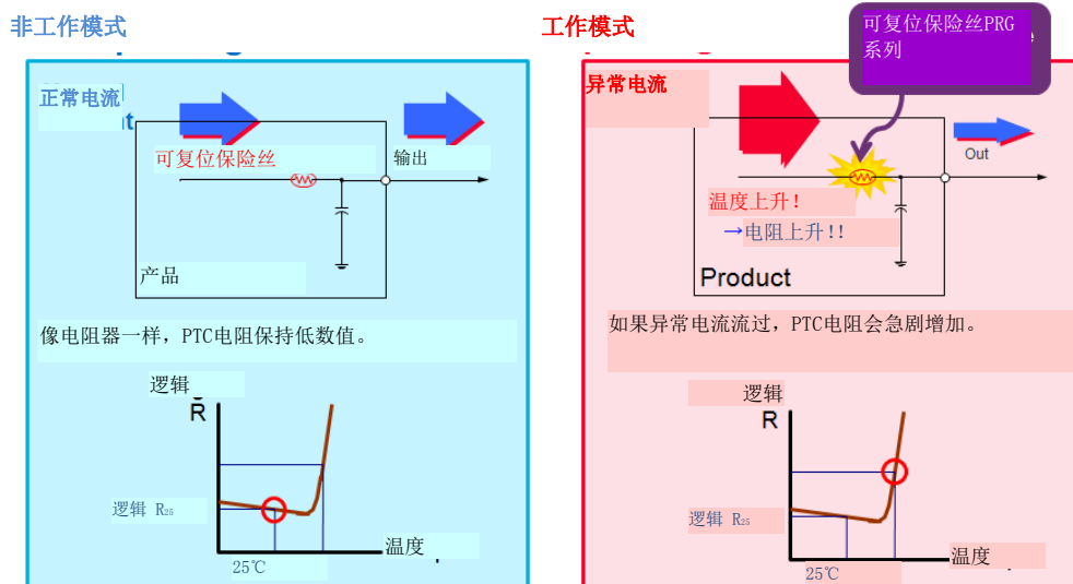
图2.2 PTC器件工作原理
