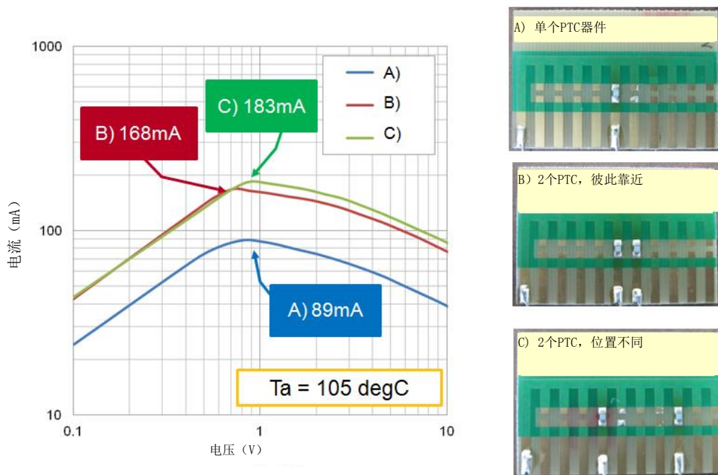
图2.8 PTC位置的影响
