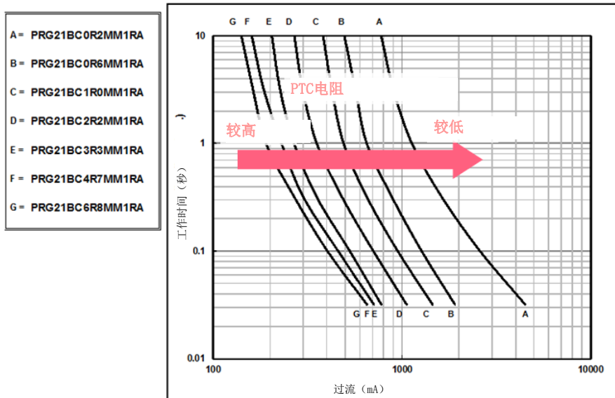
图2.9 时间跳闸动作取决于单个PTC电阻 (例如: PRG21BC*****RA 系列)
