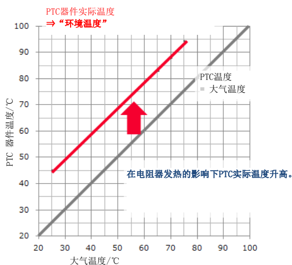
图2.6 PTC器件实际温度和大气温度
