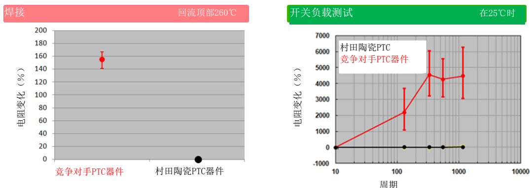
图1.4 村田陶瓷PTC与竞争对手PTC器件的比较
