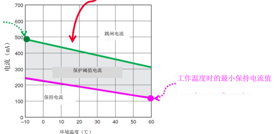
图2.4 保持电流和跳闸电流的选择过程 (例如PRG21BC3R3型)
