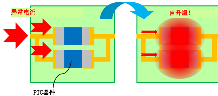
图2.7 每个PTC器件相互升温
