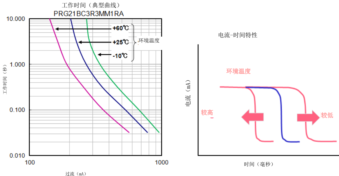
图2.10 时间跳闸动作取决于环境温度 (例如: PRG21BC3R3MM1RA)
