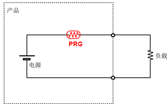
图2.1 采用PTC器件的基本电路
