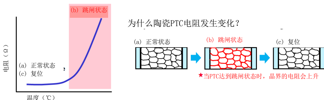
图1.1 PTC耐温特性及其起源
