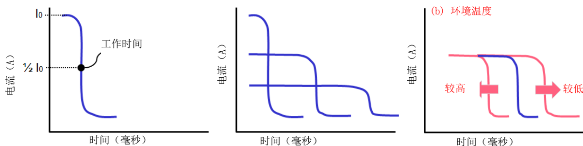
图1.3 电流-时间特性
