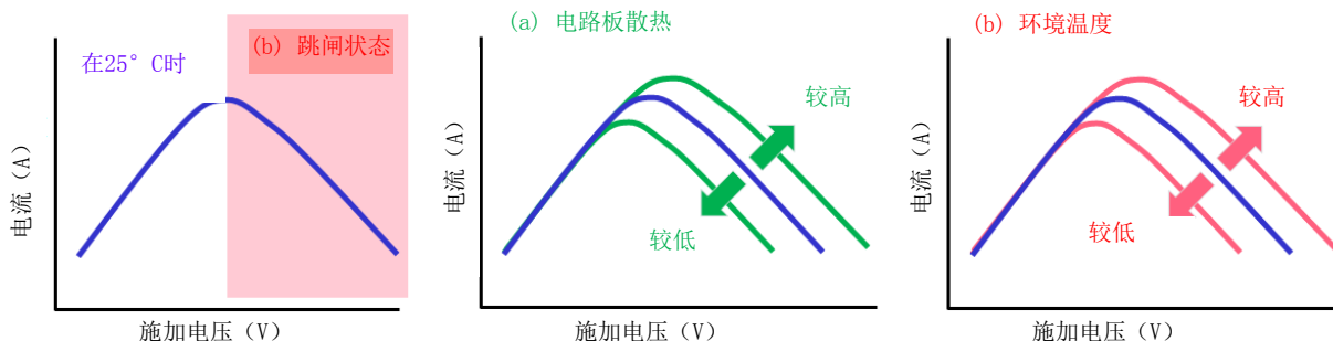
图1.2 电流-电压，取决于散热和环境温度。
