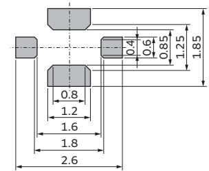
NFM21PS
