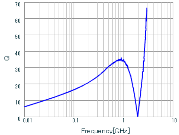
LQG15WZ51NG02 Q.
