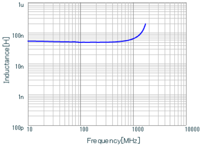
LQG15WZ51NG02 L.
