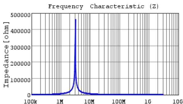
LQH43NH102J03 |Z|
