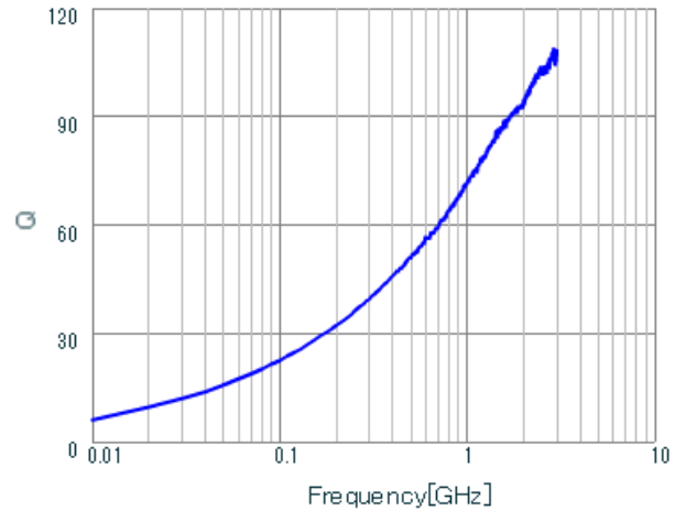
LQW15AN9N5G0Z Q.
