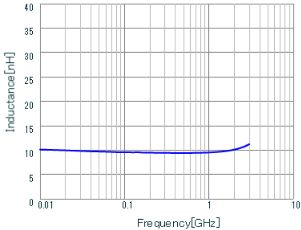
LQW15AN9N5G0Z L.
