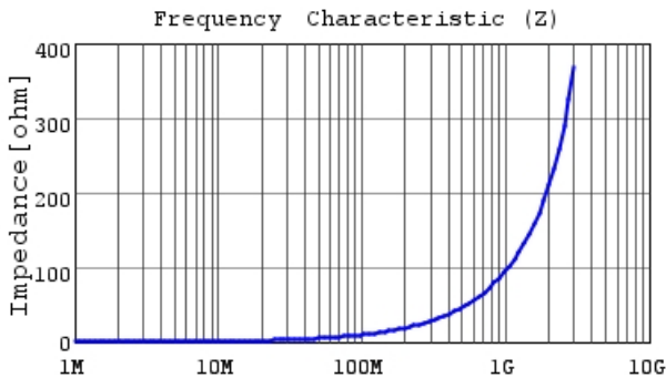
LQW18AN15NJ80 |Z|
