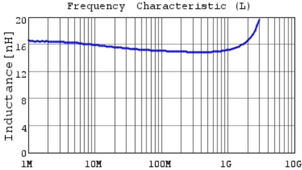
LQW18AN15NJ80 L
