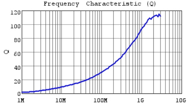
LQW18AN15NJ80 Q
