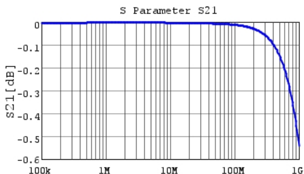
■ RHEL81H684K2M1H03A S21 DCOV, 25degC
