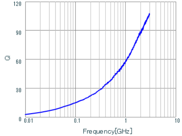
LQG15HN1N2S02 Q.
