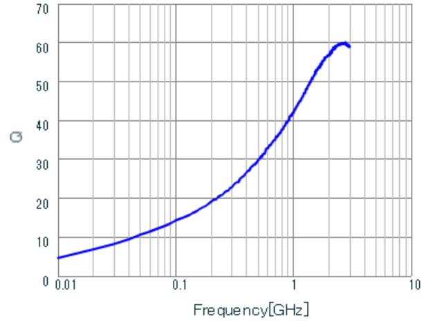
LQG15HN2N4S02 Q.
