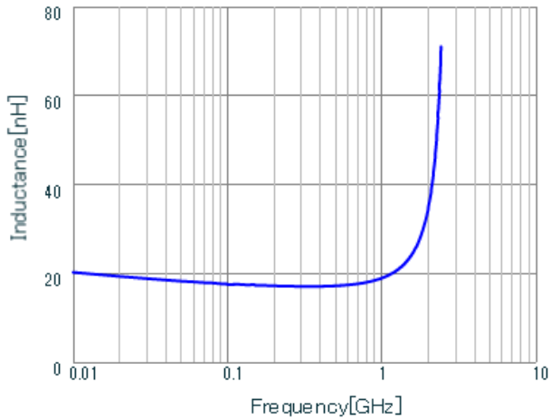
LQG15HS18NH02 L.
