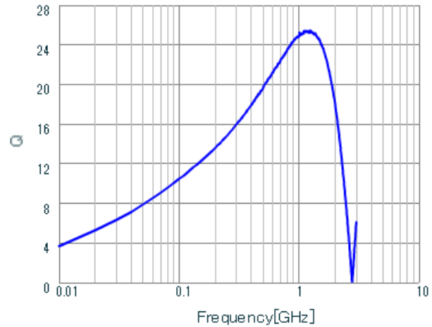
LQG15HS18NH02 Q.
