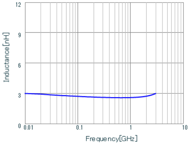
LQG15HS2N7S02 L.
