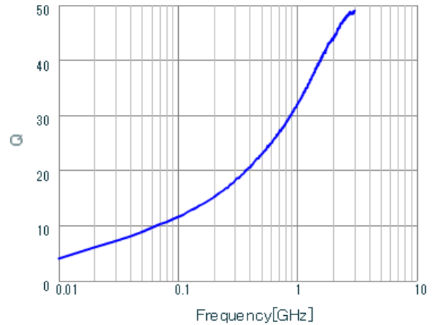
LQG15HS2N7S02 Q.
