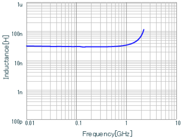
LQG15WH30NG02 L.
