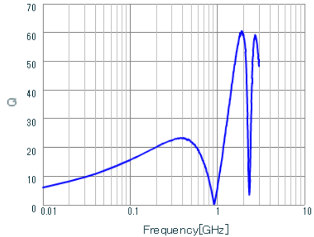
LQG18HNR10J00 Q.
