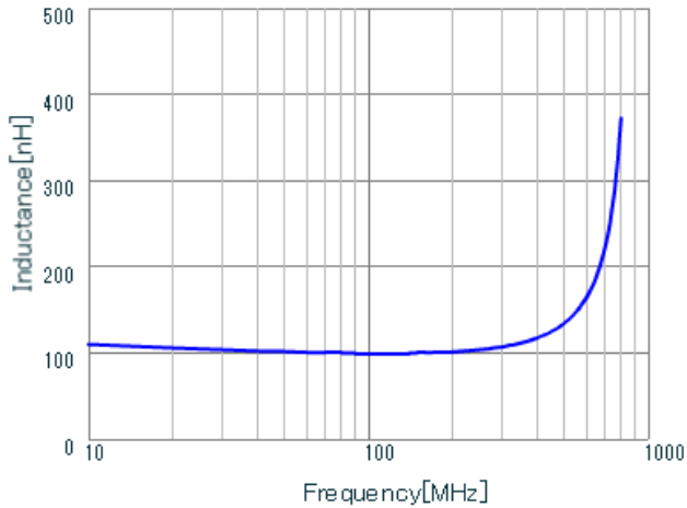
LQG18HNR10J00 L.
