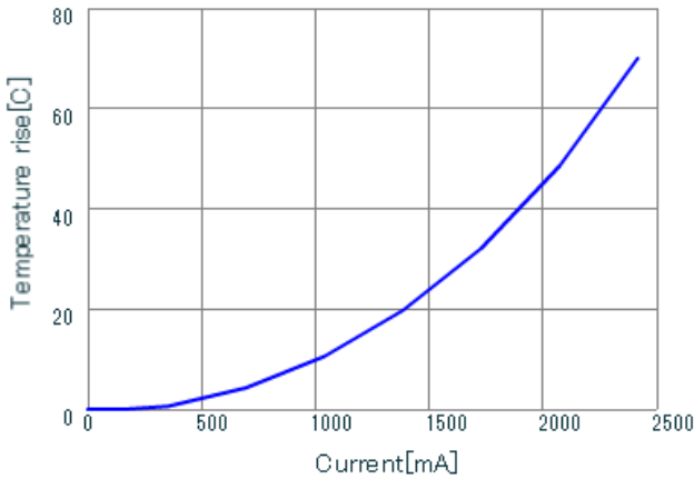
LQH2HPN2R2MJR DT_Current
