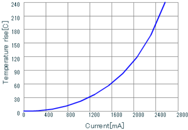
LQH3NPZ6R8MGR DT_Current
