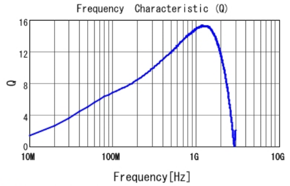
■ LQP02HQ43NJ02 Q
