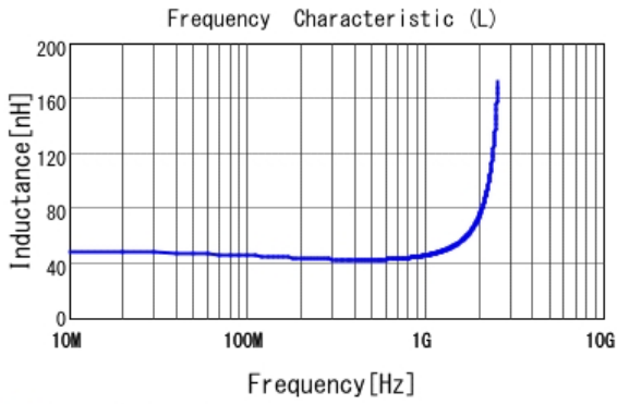
■ LQP02HQ43NJ02 L
