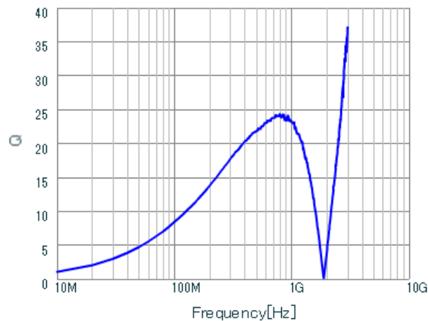
LQP03HQ68NH02 Q.
