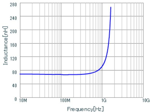
LQP03HQ68NH02 L.
