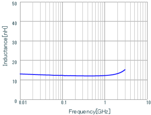
LQW15AN12NJ00 L.
