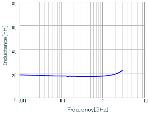
LQW15AN18NJ00 L.
