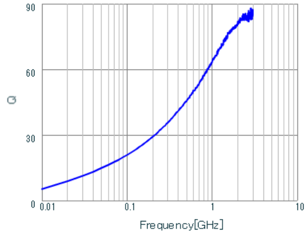
LQW15AN18NJ00 Q.
