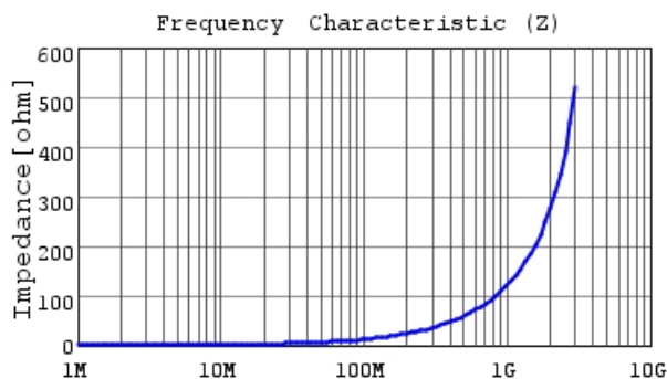
LQW15AN19NJ80 |Z|
