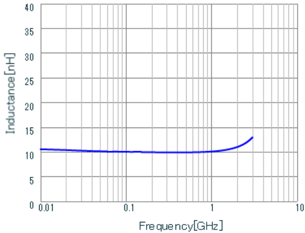
LQW18AN10NG00 L.
