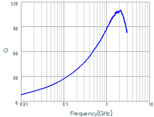
LQW18AN10NG00 Q.
