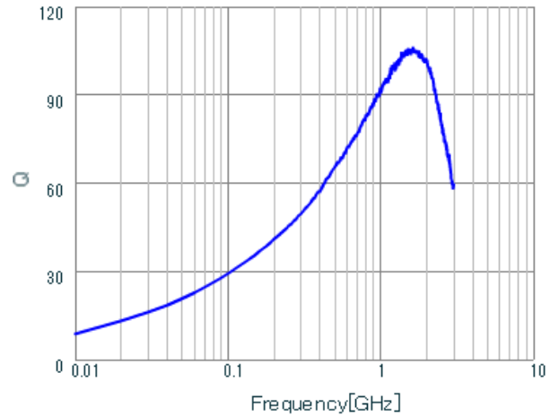
LQW18AN15NG0Z Q.
