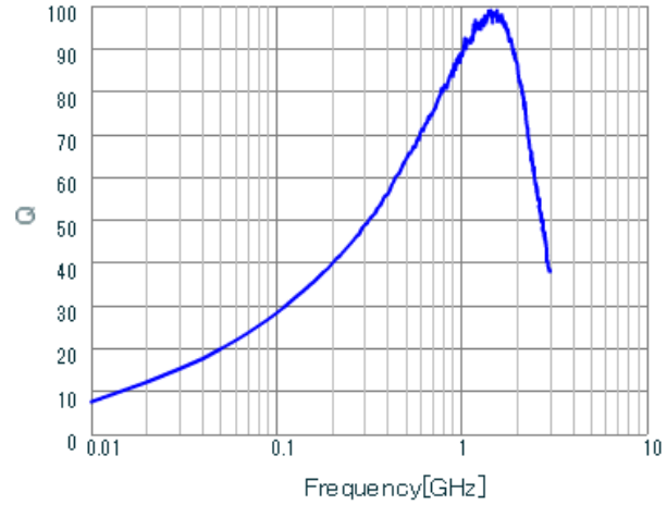
LQW18AN24NG0Z Q.
