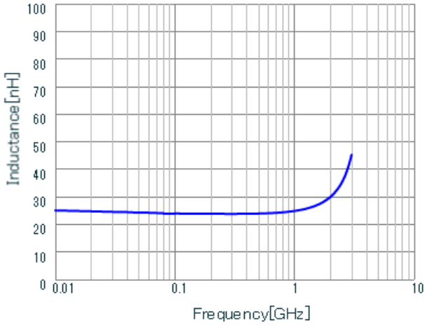
LQW18AN24NG0Z L.
