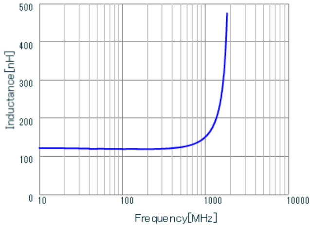
LQW18ANR12J00 L.
