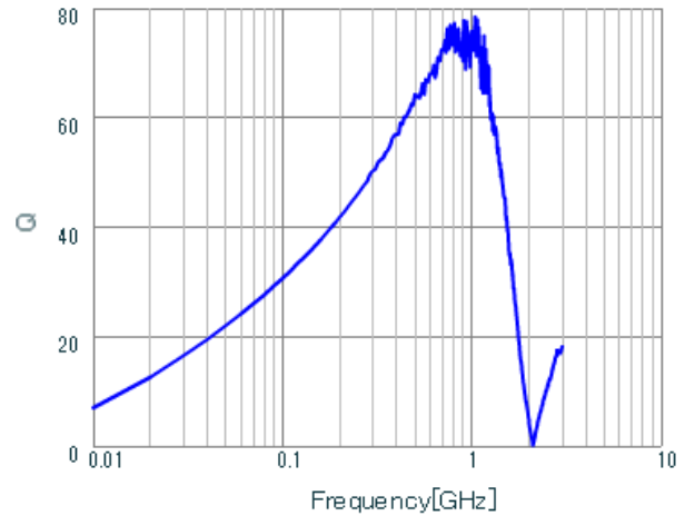
LQW18ANR12J00 Q.
