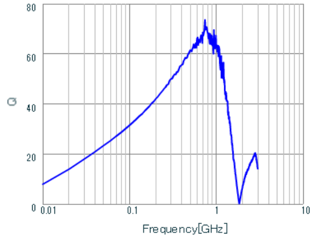
LQW18ANR15G00 Q.
