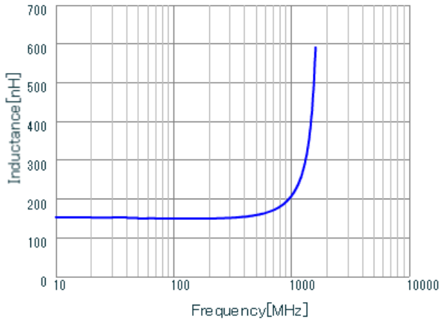
LQW18ANR15G00 L.
