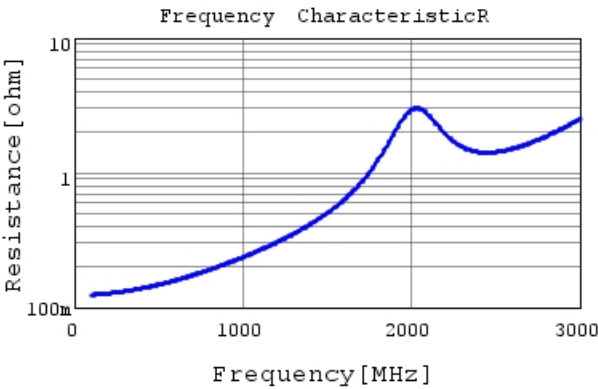
GA342A1XGF680JW31 R DCOV, 20degC
