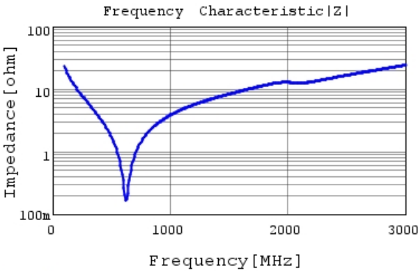
GA342A1XGF680JW31 |Z| DCOV, 20degC
