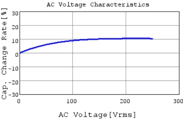
GA342A1XGF680JW31 C-AC Voltage capchange, D
