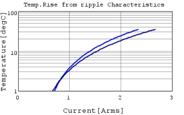
GRM155R60J474KE19 Temp.rise — 500kHz —
