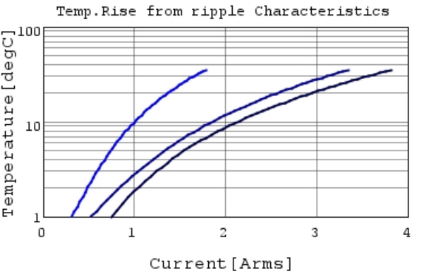
GRM188R60J105KA01 Temp.rise 100kHz
