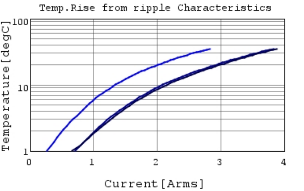
GRT155R60J475ME13 Temp.rise — 100kHz —
