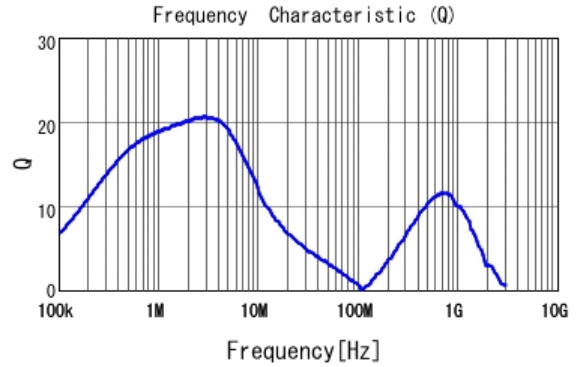
■ 1226AS-H-2R7M Q
