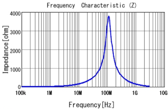
■ 1226AS-H-2R7M |Z|
