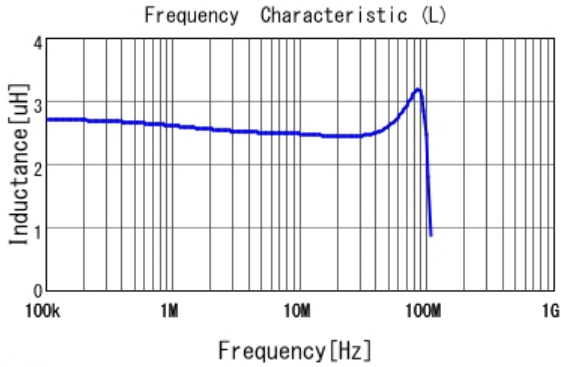
■ 1226AS-H-2R7M L
