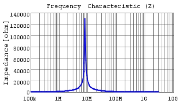
LQH43NH181J03 |Z|
