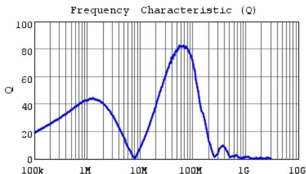
LQH43NH181J03 Q
