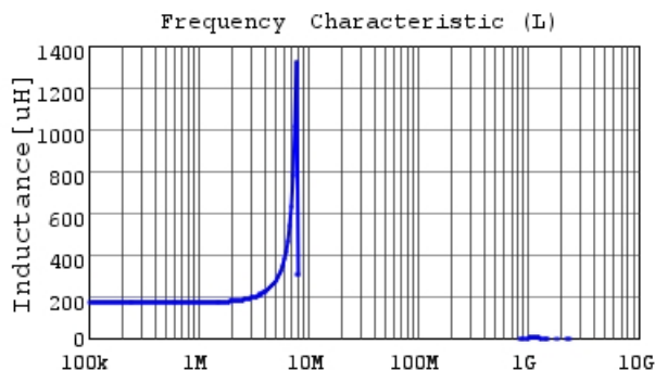
LQH43NH181J03 L
