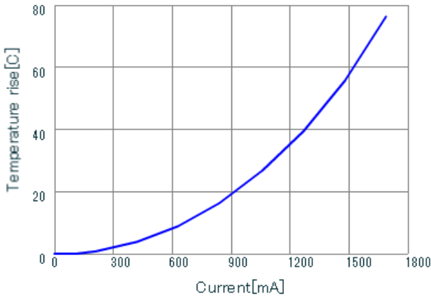
LQH44PZ100MGR DT_Current
