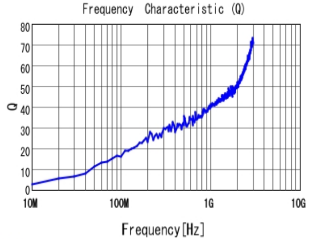
■ LQP02HQ0N4C02 Q
