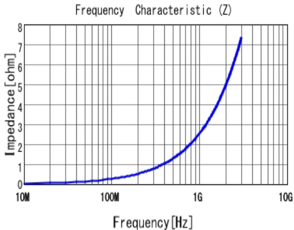
■ LQP02HQ0N4C02 |Z|
