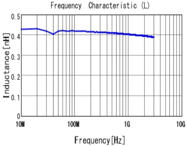
■ LQP02HQ0N4C02 L
