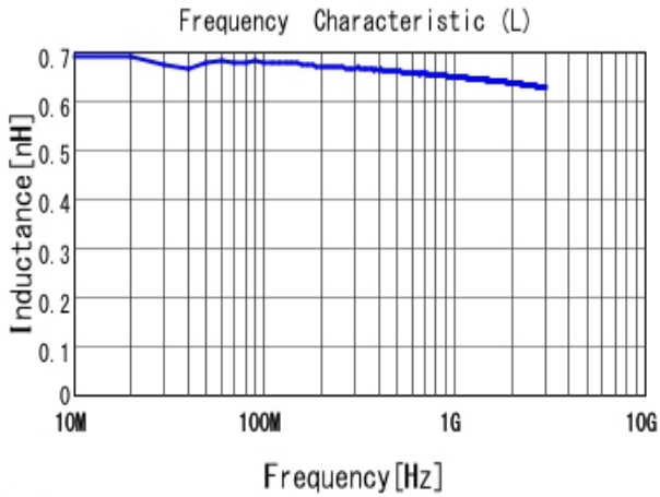
■ LQP02HQ0N6B02 L
