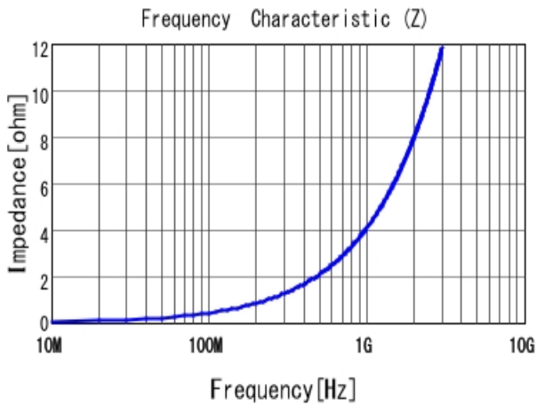
■ LQP02HQ0N6B02 |Z|
