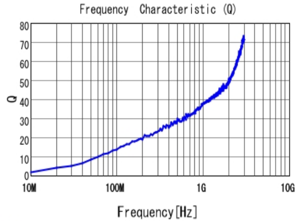
■ LQP02HQ0N6B02 Q
