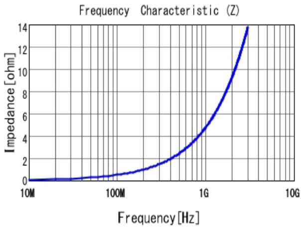
■ LQP02HQ0N8B02 |Z|
