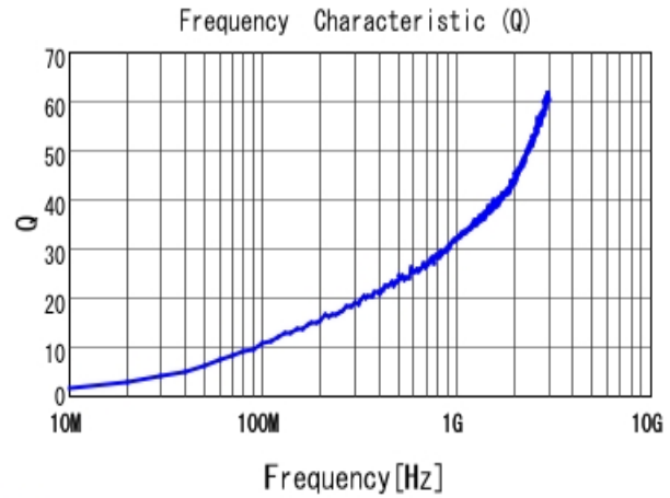
■ LQP02HQ0N8B02 Q
