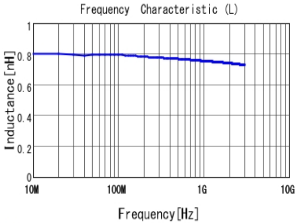
■ LQP02HQ0N8B02 L
