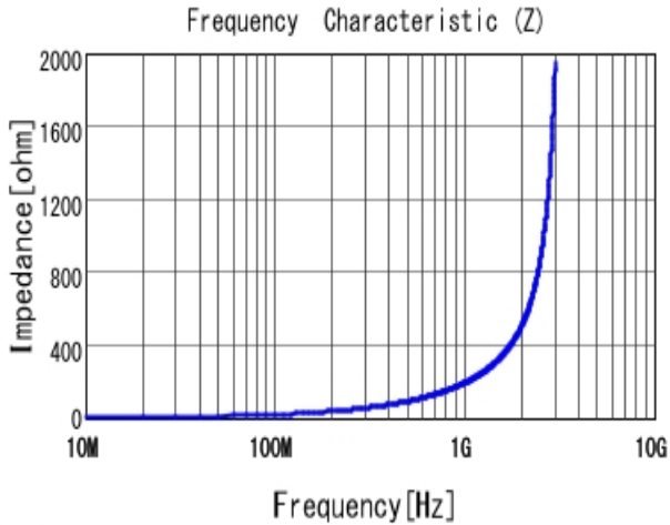
■ LQP02HQ33NJ02 |Z|
