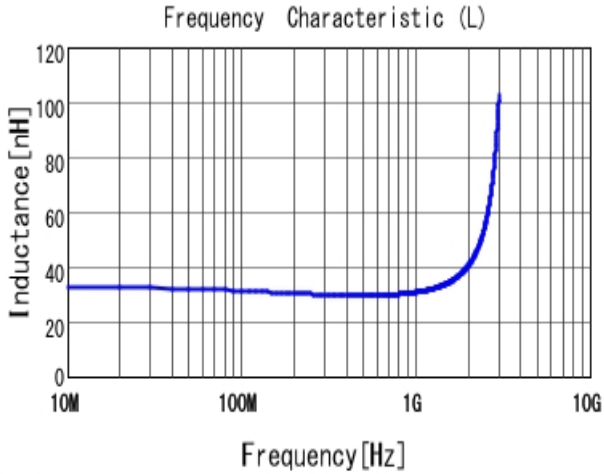
■ LQP02HQ33NJ02 L
