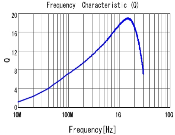
■ LQP02HQ33NJ02 Q
