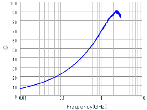
LQW15AN15NJ00 Q.
