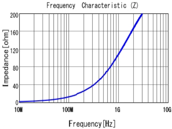
■ LQW15CA22NJ00 |Z|
