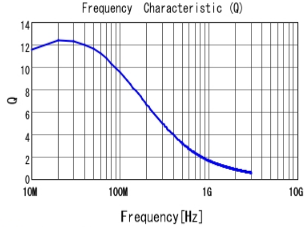
■ LQW15CA22NJ00 Q
