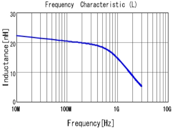
■ LQW15CA22NJ00 L
