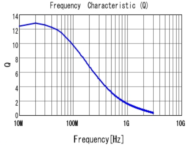
■ LQW15CA39NJ00 Q
