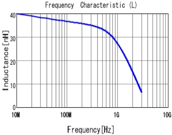
■ LQW15CA39NJ00 L
