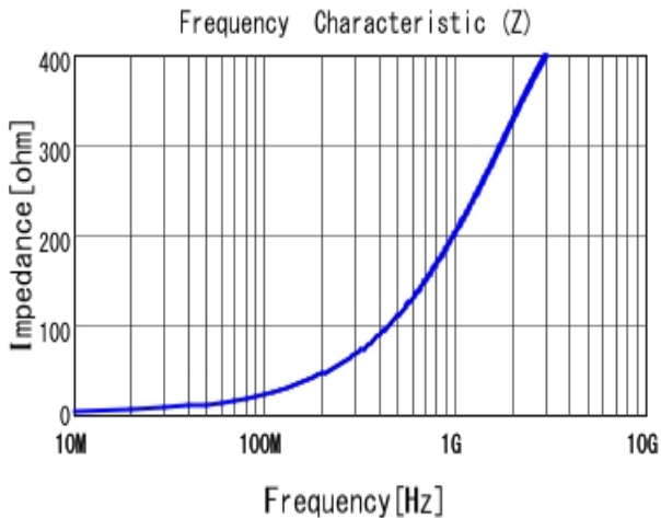
■ LQW15CA39NJ00 |Z|
