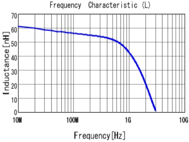
■ LQW15CA59NJ00 L
