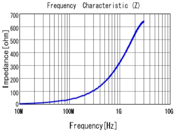
■ LQW15CA59NJ00 |Z|
