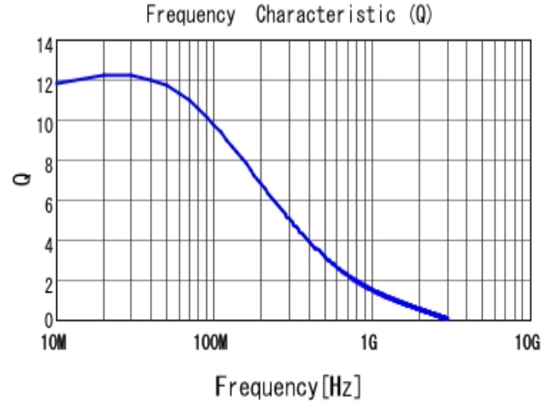
■ LQW15CA59NJ00 Q
