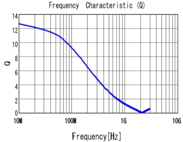
■ LQW15CAR11J00 Q
