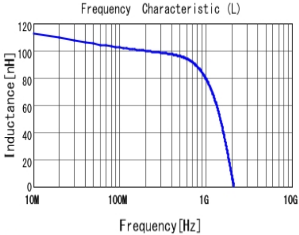
■ LQW15CAR11J00 L
