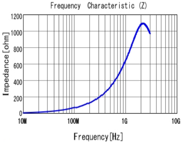
■ LQW15CAR11J00 |Z|
