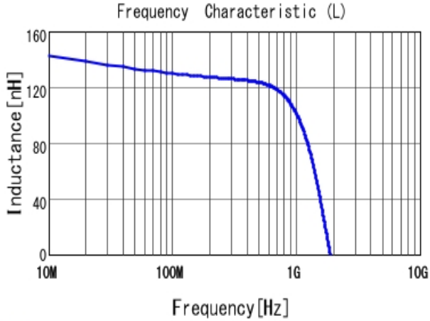
■ LQW15CAR14J00 L
