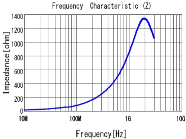
■ LQW15CAR14J00 |Z|
