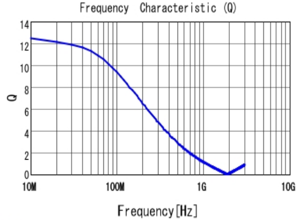
■ LQW15CAR14J00 Q
