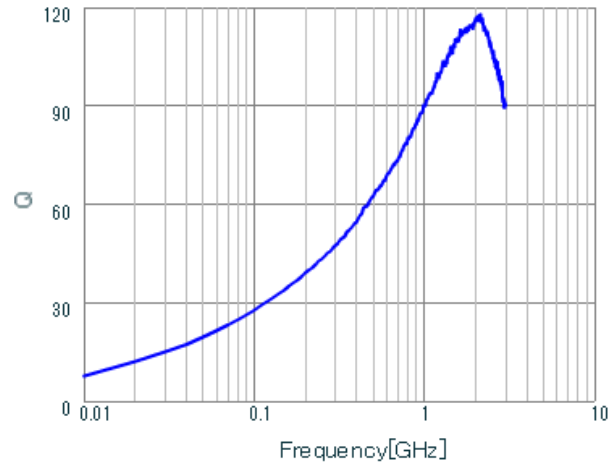
LQW18AN12NG0Z Q.
