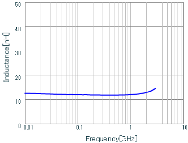
LQW18AN12NG0Z L.
