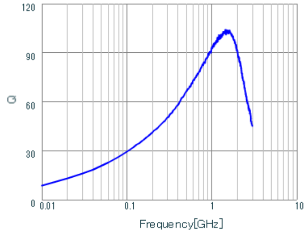
LQW18AN22NG0Z Q.
