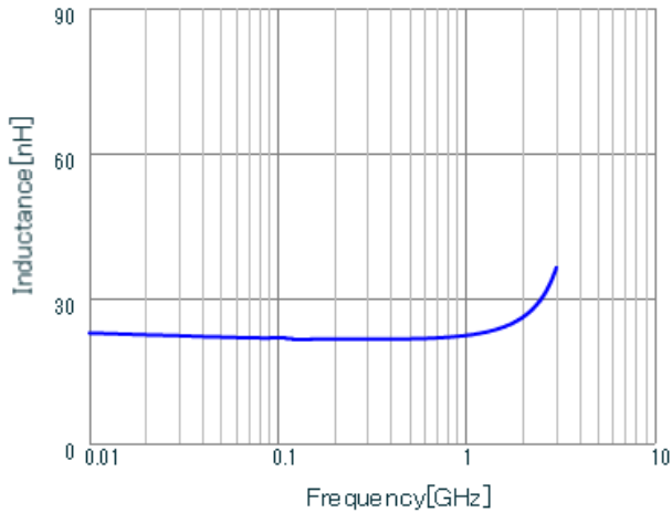
LQW18AN22NG0Z L.
