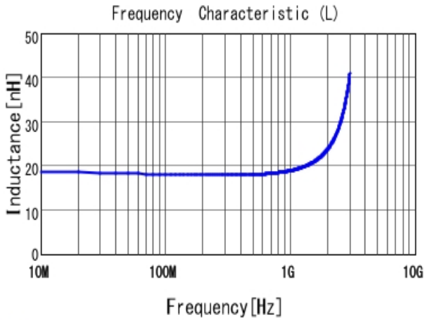
■ LQW2BAS18NJ00 L
