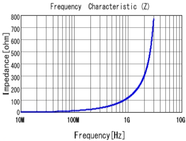
■ LQW2BAS18NJ00 |Z|
