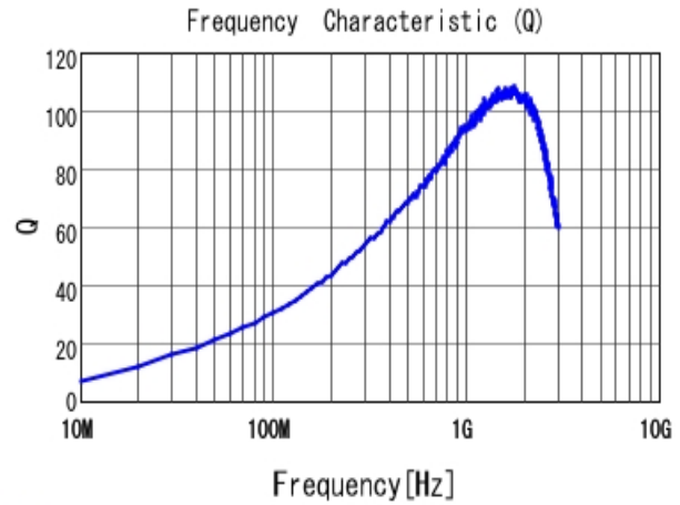
■ LQW2BAS18NJ00 Q
