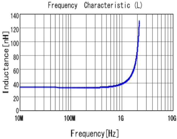
■ LQW2BAS33NJ00 L
