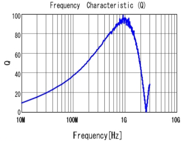
■ LQW2BAS33NJ00 Q
