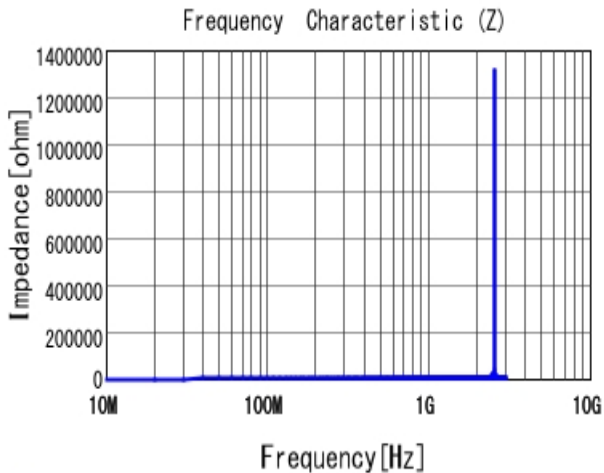
■ LQW2BAS33NJ00 |Z|
