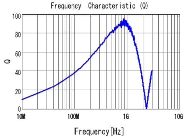
■ LQW2BAS36NG00 Q
