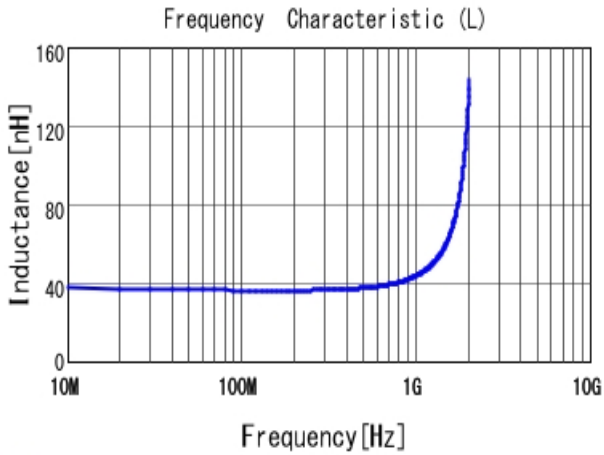
■ LQW2BAS36NG00 L
