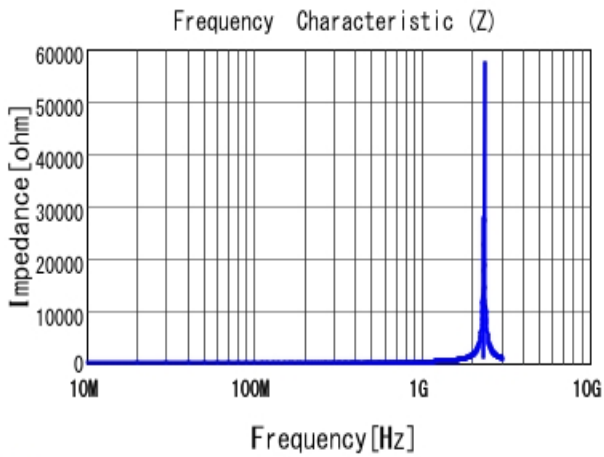
■ LQW2BAS36NG00 |Z|
